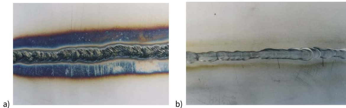
3. ábra. A gyökoldal formálógáz (a) és anélküli (b) kialakításával készített varrat összehasonlítása
